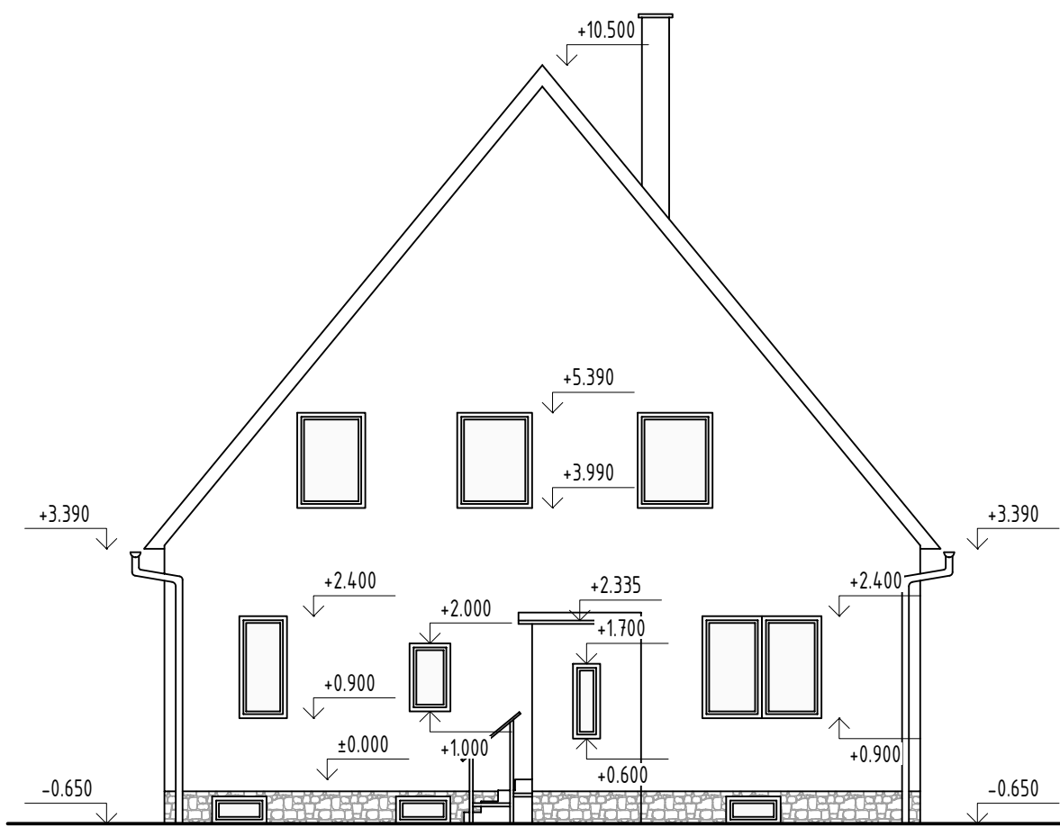
POHLED SEVERNÍ
