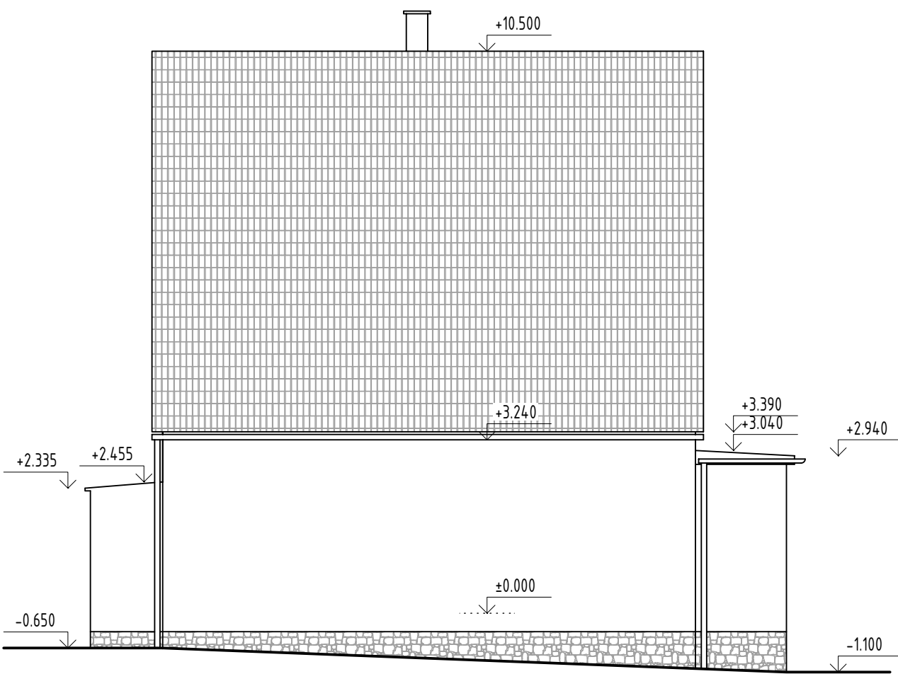
POHLED ZÁPADNÍ
