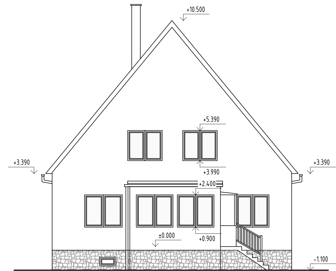
POHLED JIŽNÍ
