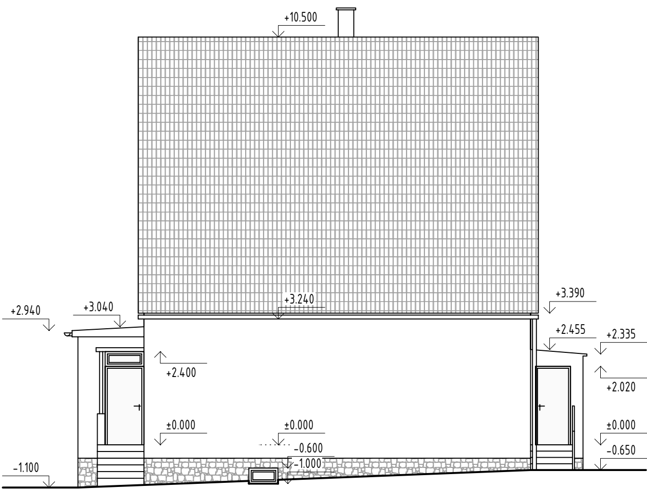
POHLED VÝCHODNÍ
